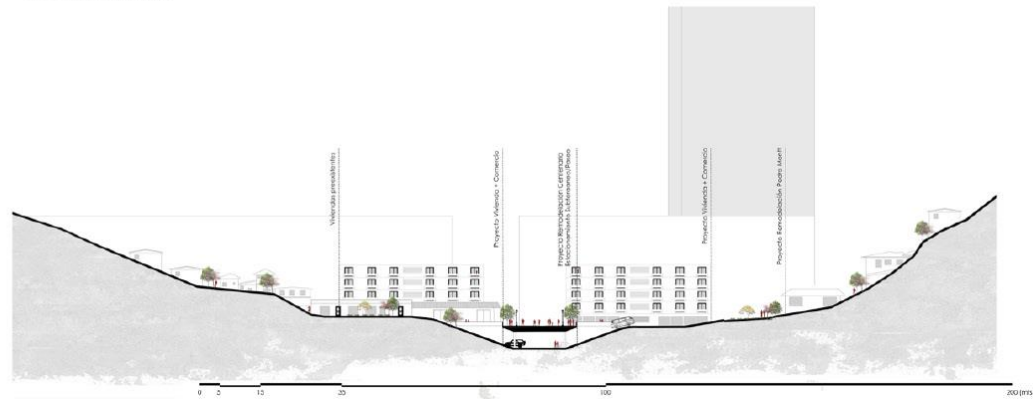
CORTE FF' CENTENARIO TRANSVERSAL
